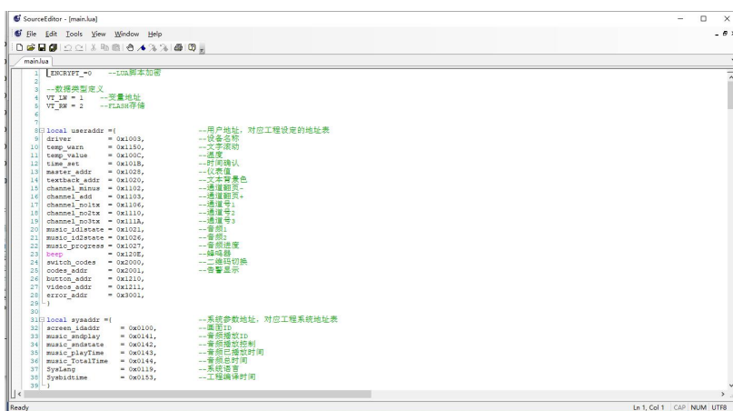
图 10-2 LUA 脚本编辑器
